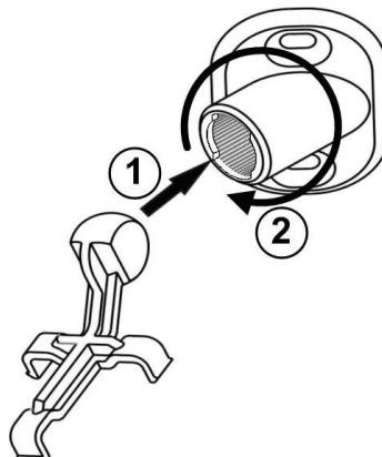
Рис.10 Схема соединения кронштейна и держателя
